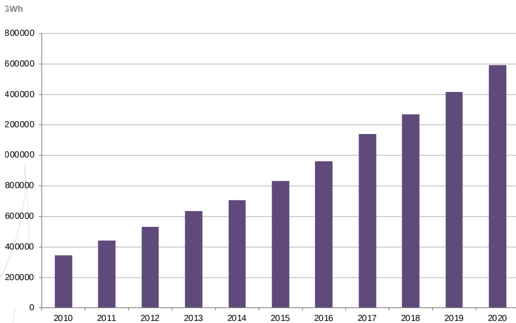
Produzione eolica lorda a livello mondiale (2010-2020)
